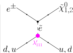
Gaugino production
